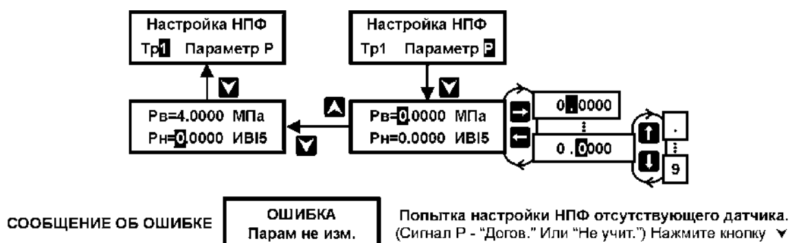
Рисунок 6.2 – Последовательность действий по настройке НПФ датчиков давления
