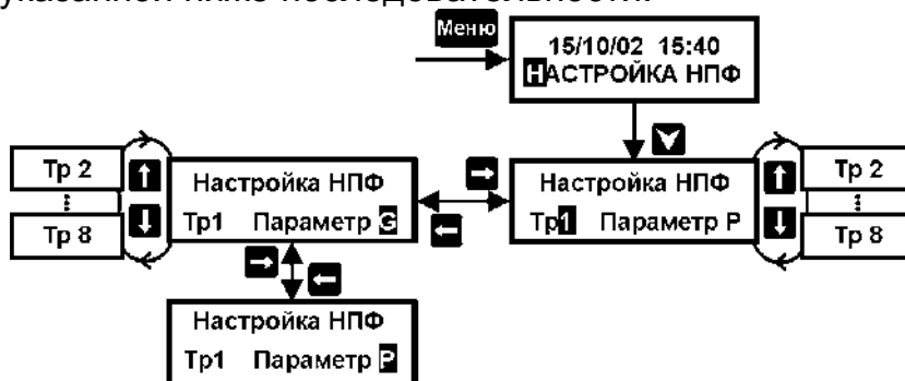
Рисунок 6.1 – Последовательность действий по настройке НФП датчиков давления и расхода.
