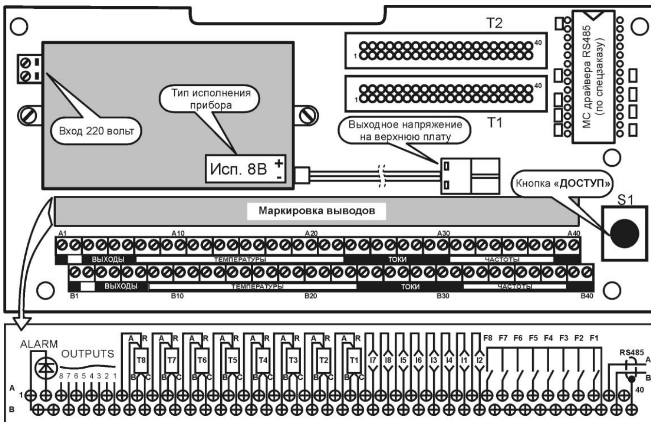
Рисунок 2 – Внешний вид платы клеммников
