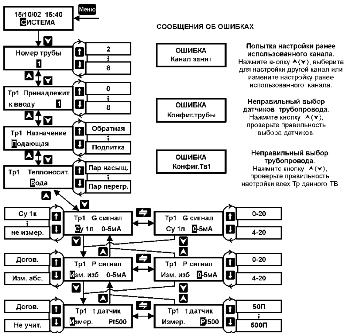
Рисунок 4 – Последовательность действий при настройке конфигурации системы
