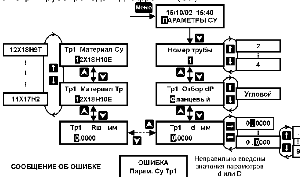
Рисунок 5 – Последовательность действий по установке параметров СУ
