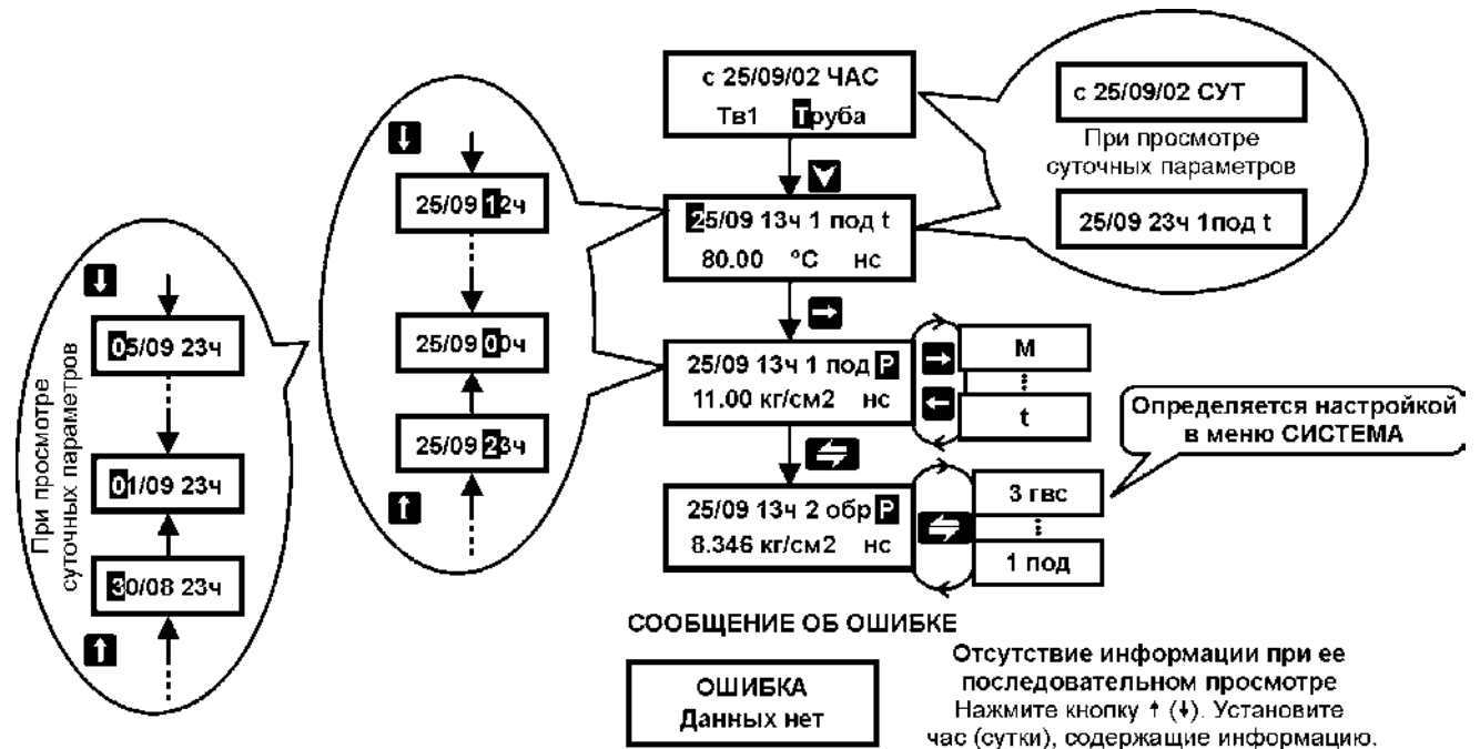
Рисунок 21 – Просмотр архивной информации по трубопроводу
