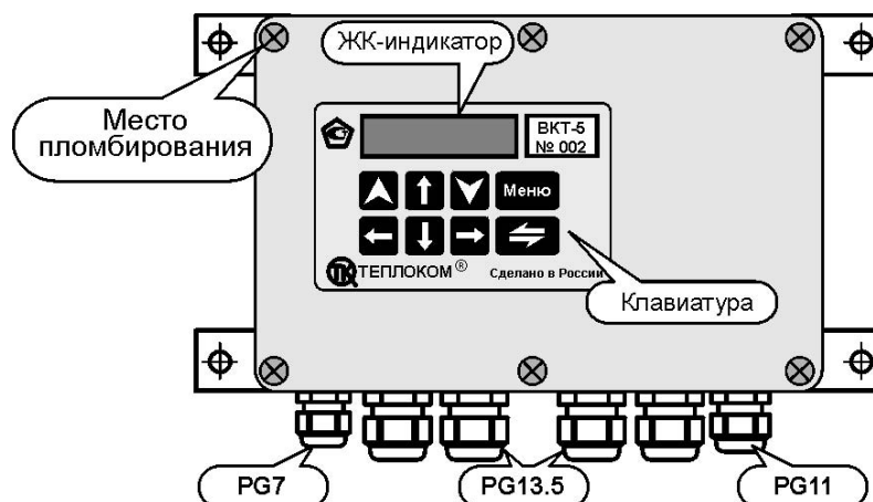
Рисунок 1 – Внешний вид вычислителя
