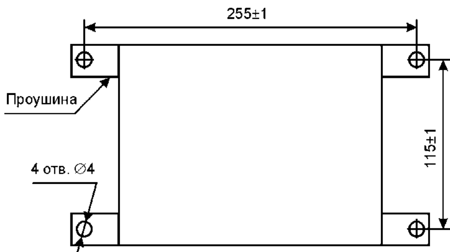
Рисунок 16 – Присоединительные размеры вычислителя
