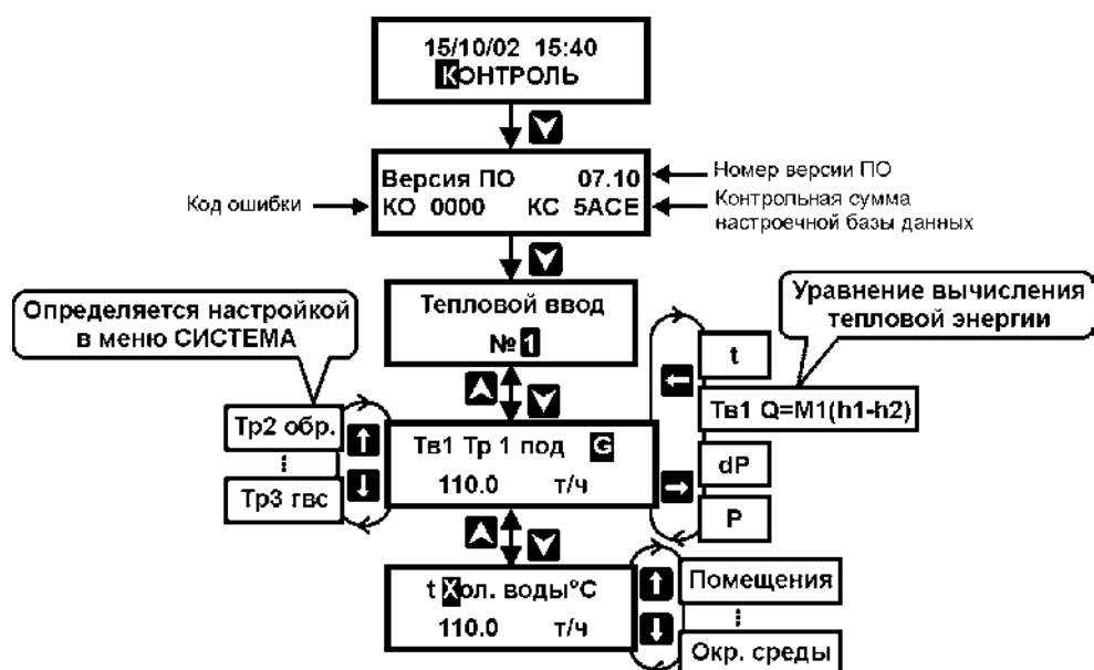
Рисунок 17 – Порядок действий по просмотру текущих параметров теплоносителя
