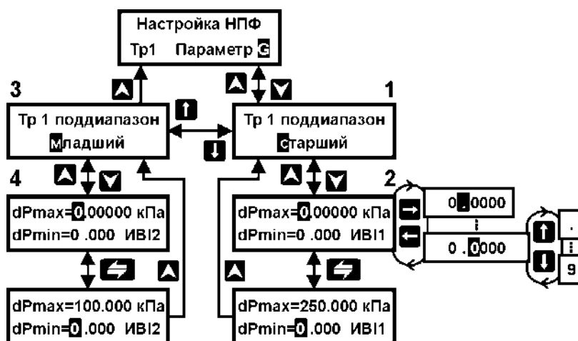
Рисунок 6.5. Настройка НПФ для расходомера переменного перепада
